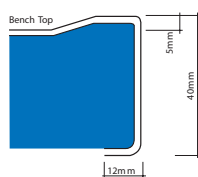
Wet edge
