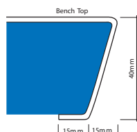
Slope edge
